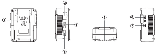
①V型卡件 ②D-TAP接口 ③USB-A接口 ④Type-C接口 ⑤BP电极接口 ⑥LED电量指示灯 ⑦电量显示按钮
